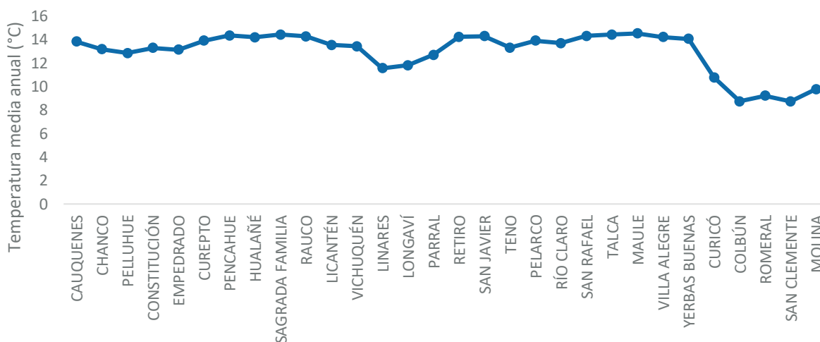
Figura 6. Temperatura media anual para la región del Maule
