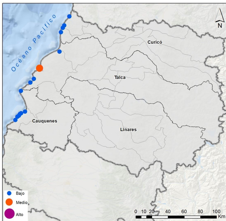
Figura 20. Mapa de riesgo ante marejadas para la costa de la Región del Maule.
