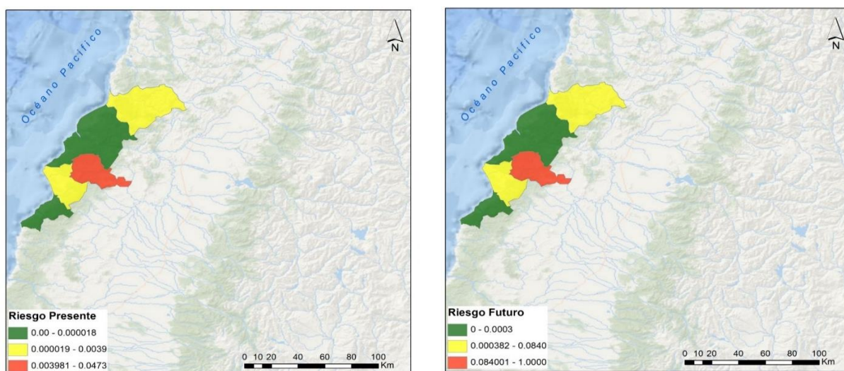
Figura 25. Índice de riesgo actual y futura para incendios en bosques de Ruil
