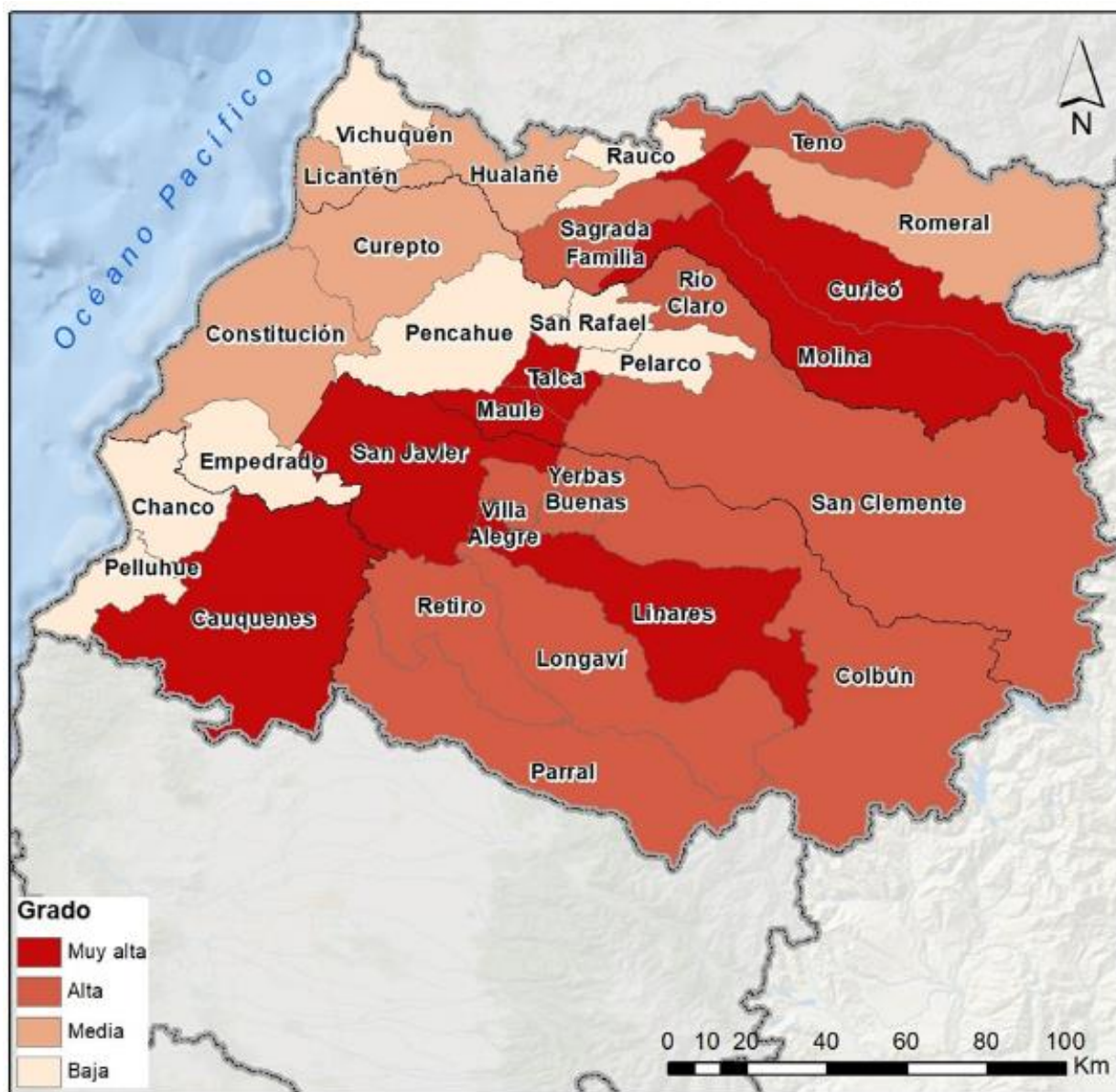
Figura 22. Mapa de caracterización de la vulnerabilidad global para la Región del Maule
